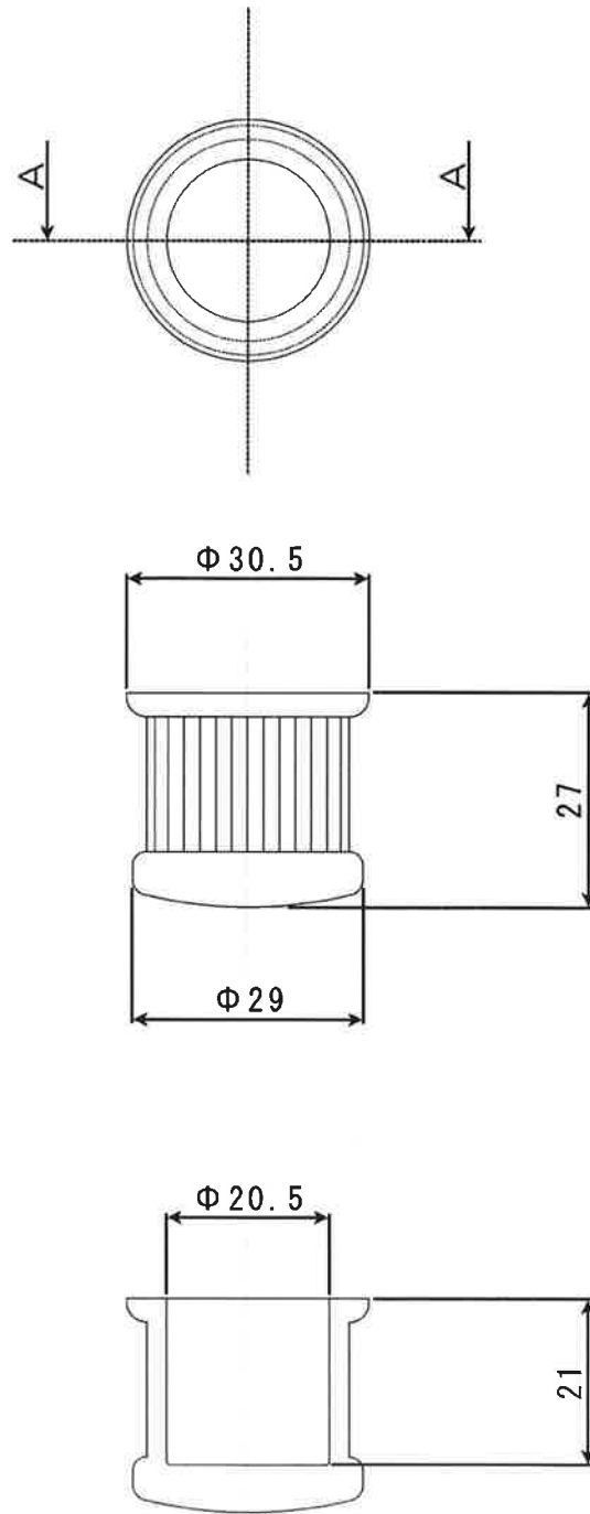
A-A断面
