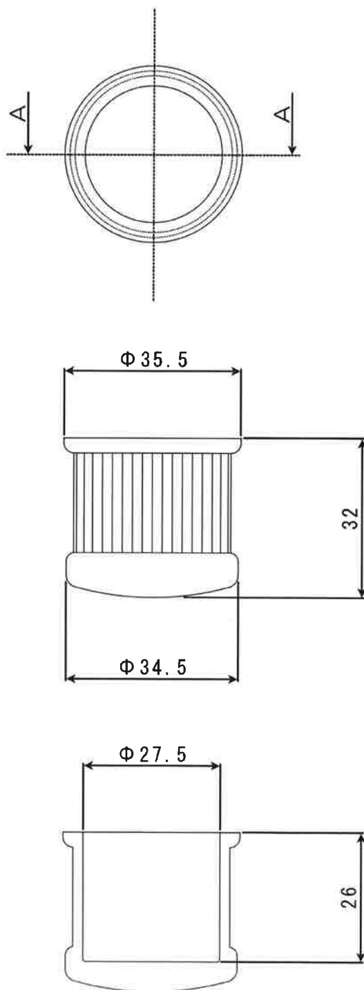
A-A断面
