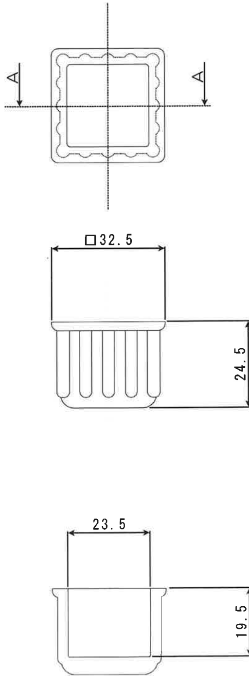
A-A断面
